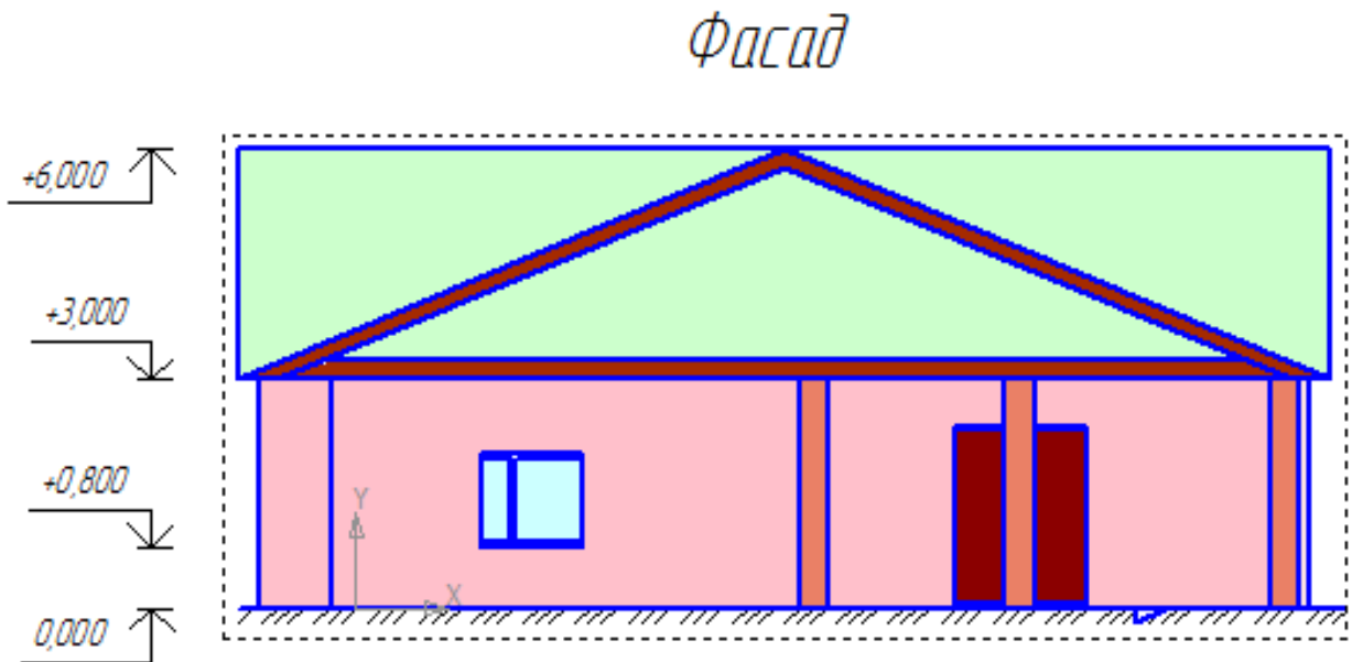
Рисунок 3.1.6. Оформление фасада
