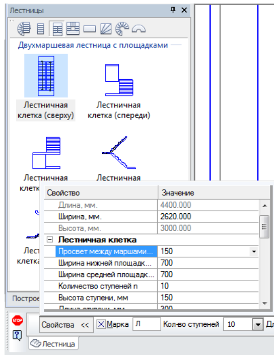
Рисунок 1.4.9. Параметры двухмаршевой лестницы.
