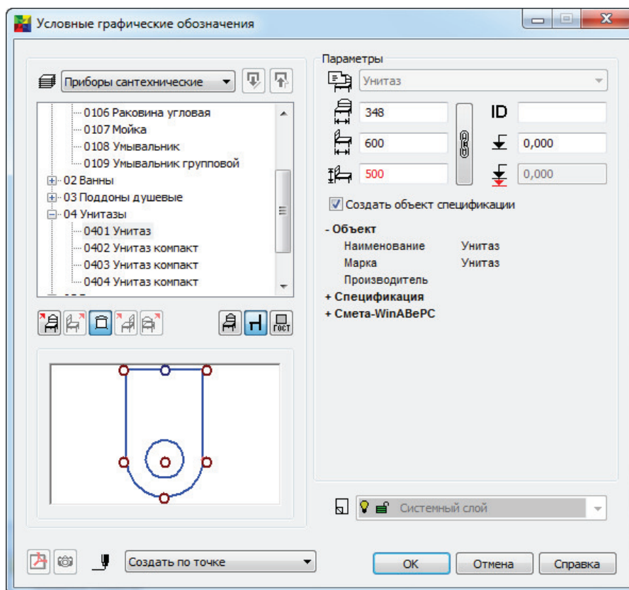
Опции диалога
