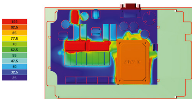
Температура поверхности компонентов платы, °C
